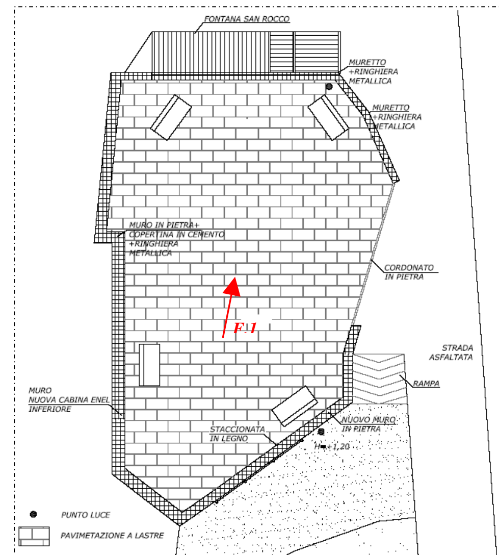
PLANIMETRIA GENERALE
