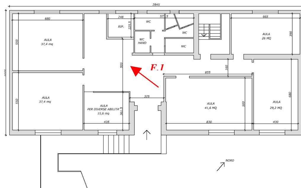
PIANTA PIANO TERRA - prima dell'intervento
